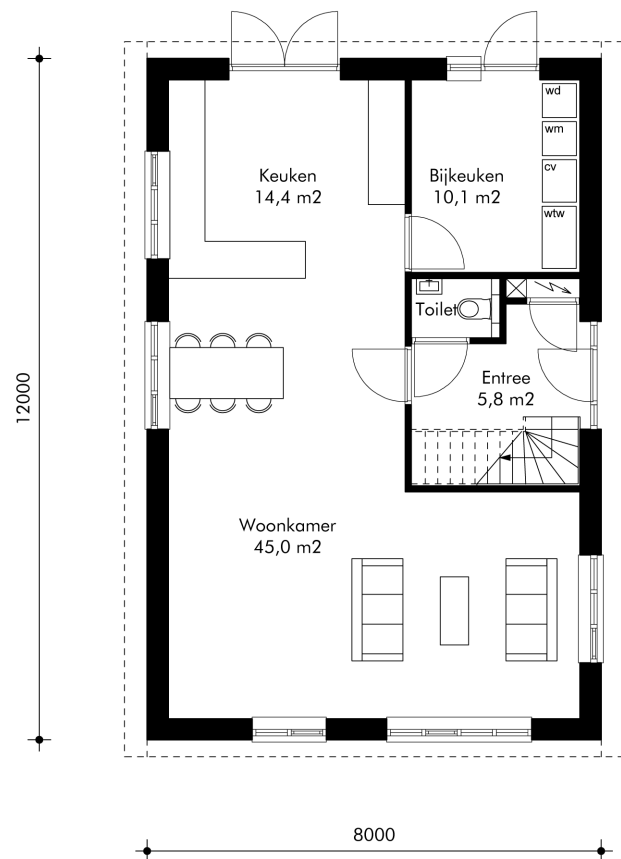
Begane grond
