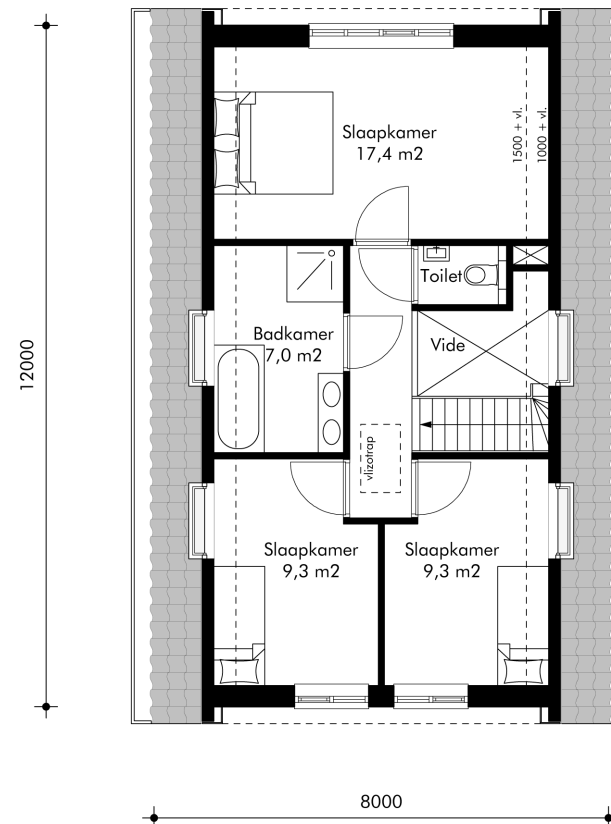
Verdieping
