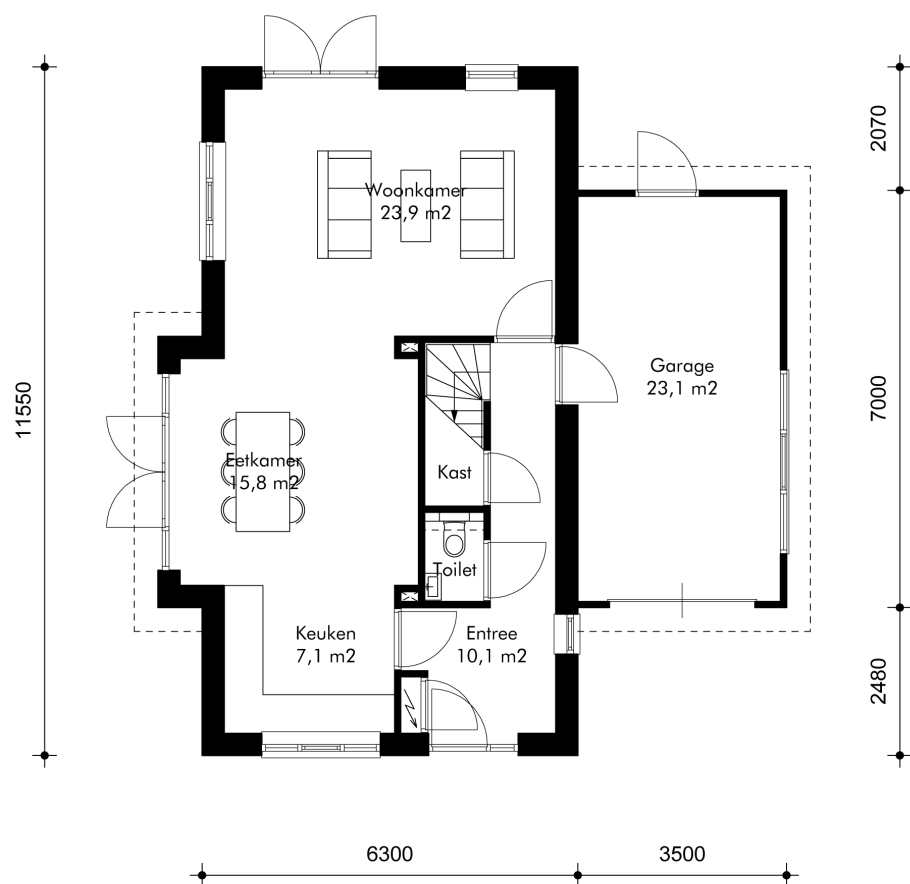
Begane grond
