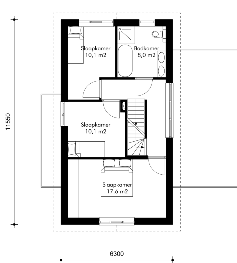
Verdieping
