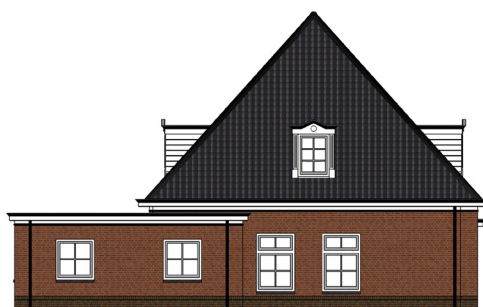
Linkergevel
